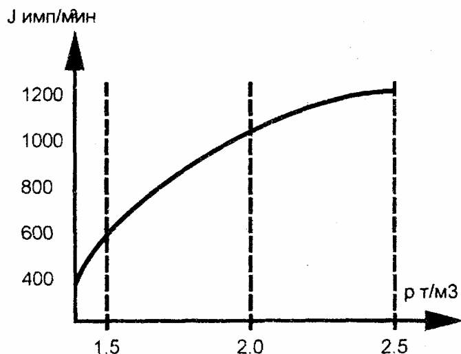
Рис. 6. Тарировочная зависимость.
