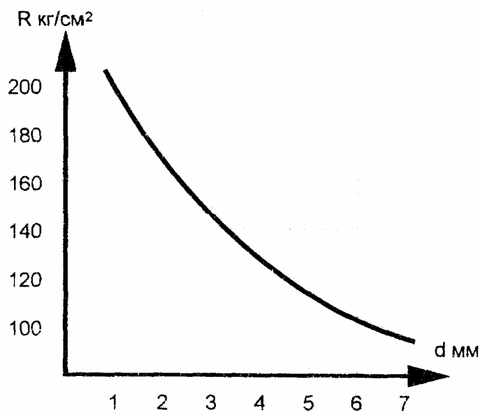
Рис.1 Тарифовочная зависимость размера отпечатка от прочности бетона
