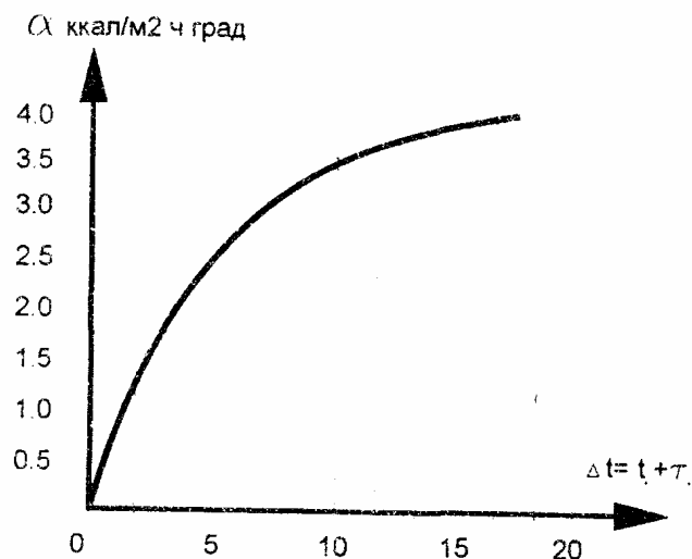
Рис.7 Определение t у вертикальных поверхностей
