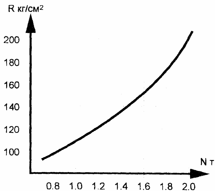
Рис.3. Тарировочная зависимость усилия вырыва от прочности бетона
