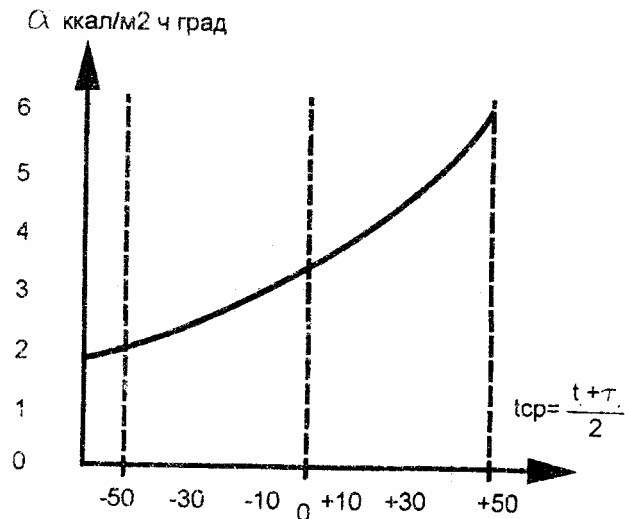
Рис.8. Определение t у вертикальных поверхностей
