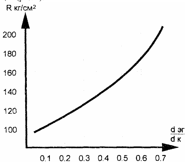
Рис. 2 Тарифовочная зависимость отношения размера отпечатка на эталоне к размеру отпечатка на поверхности конструкции от прочности бетона
