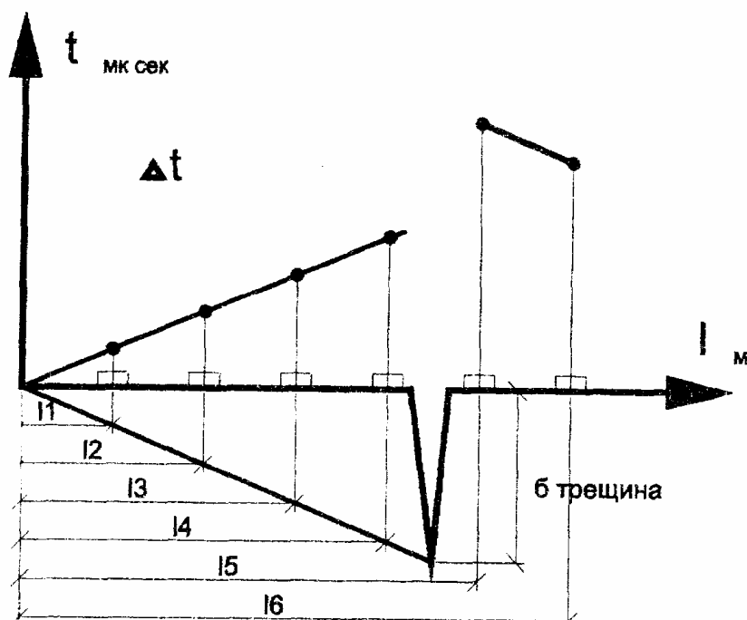
Рис. 4. Годограф при определении глубины проникания трещины
