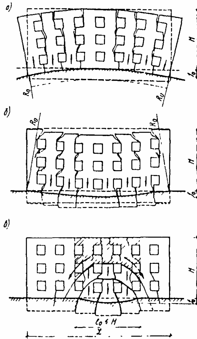
Рис. 17. Деформации и развитие трещин в стенах зданий при различных формах просадок грунта а - на длине здания z выпуклостью вверх; б - то же, вниз; в - при местной просадке грунта на длине l_0 \leq H
