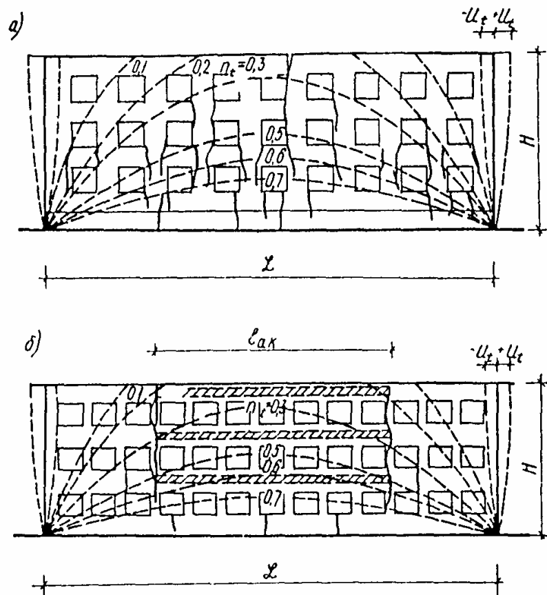
Рис. 16. Напряженное состояние ( n_i ), деформации ( U_i ) и развитие трещин в стенах каменных зданий при температурно-влажностных воздействиях а - при отсутствии продольного армирования стен (поясов); б - то же, при армировании на длине l_{ak} (заштриховано)
