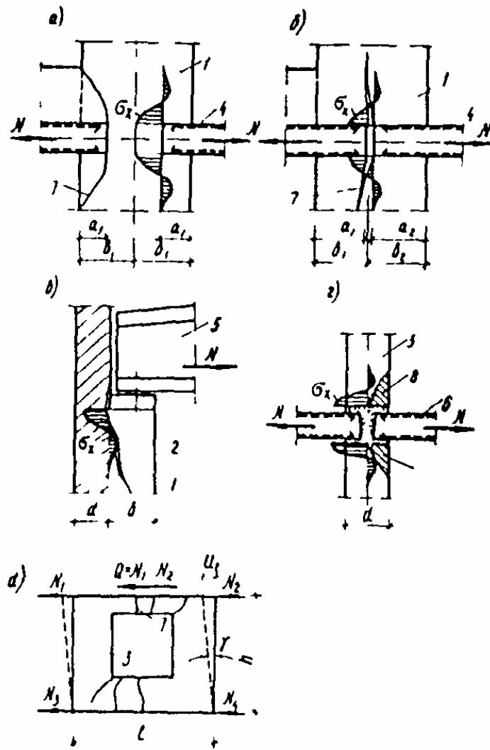
Рис. 13. Напряженное состояние ( \sigma_x ) и повреждения элементов каменных, блочных и панельных стен при действии горизонтальных сил N (температура, усадка и т.п.) а, б - простенков (блоков) при частичном ( a < e ) и сплошном ( a = e ) опирании перемычек; в - пилястр; г - стеновых панелей при платформенном опирании на перекрытие; д - то же, при растяжении и сдвиге в плоскости стены 1 - простенок (блок); 2 - пилястра; 3 - панель (блок); 4 - перемычка; 5 - балка; 6 - плита перекрытия; 7 - трещина; 8 - скол
