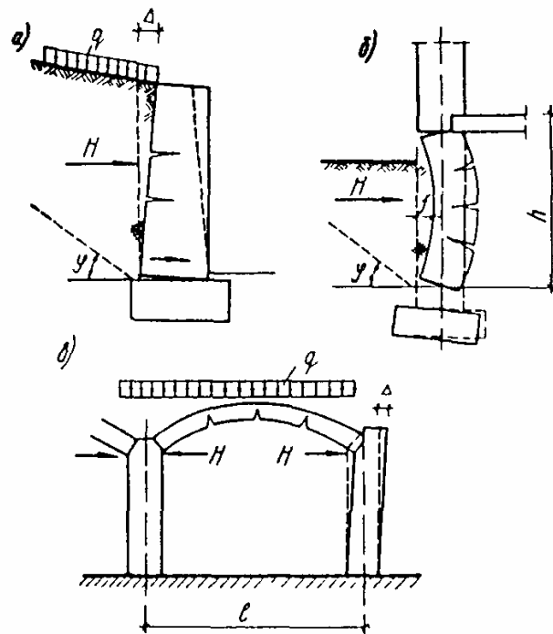
Рис. 15. Деформации и повреждения каменных конструкций при действии горизонтальных сил а - подпорная стенка; б - фундамент; в - каменный свод
