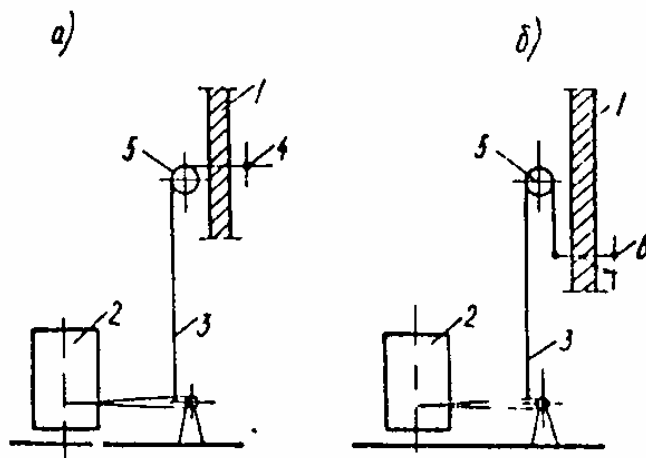
Рис. 6. Измерение раскрытия (а) и сдвига (б) по шву сборных элементов с
