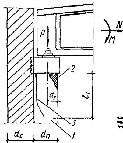
Рис. 10. Характерные случаи повреждения опорных участков пилястр каменных стен при опирании на них ферм и балок 1 - пилястра; 2 - краевое раздробление и сколы кладки под опорой; 3 - вертикальные трещины
