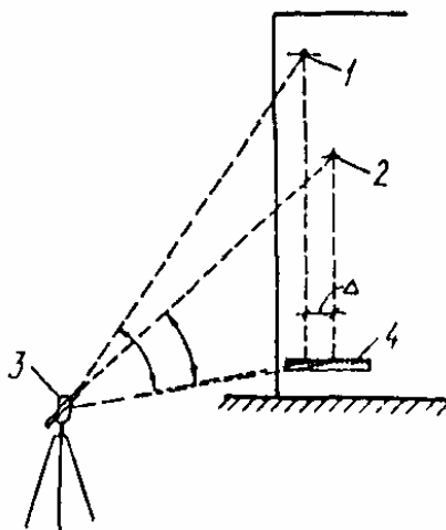
Рис. 1. Измерение горизонтального смещения, двух точек (1 и 2) стены здания методом сноса вертикали с помощью теодолита 1, 2 - точки; 3 - теодолит; 4 - переносная линейка с миллиметровыми делениями
