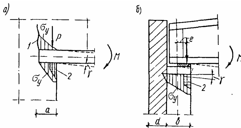
Рис. 11. Напряженное состояние ( \sigma_y ) и повреждения кладки опор перемычек и балок при изгибе ( \gamma ) и внецентренном сжатии ( e ) а - при заделке в кладку; б - то же, при опирании 1 - трещина; 2 - раздробление кладки
