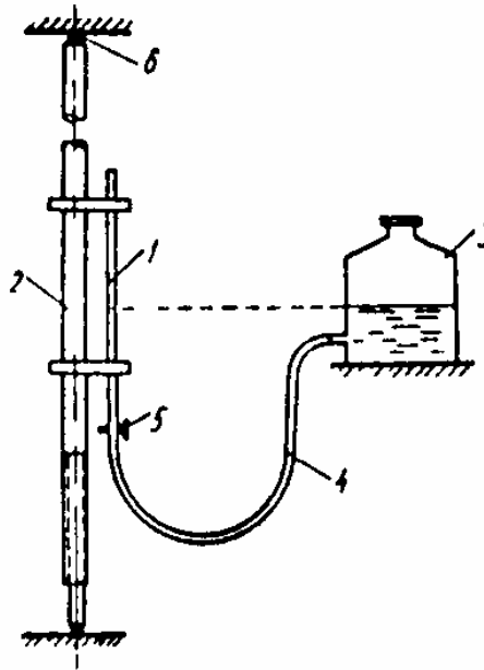
Рис. 5. Схема измерения прогибов перекрытий гидростатическим уровнем 1 - градуированная трубка; 2 - телескопическая стойка; 3 - сосуд; 4 - резиновый шланг; 5 - краник; 6 - точка измерения
