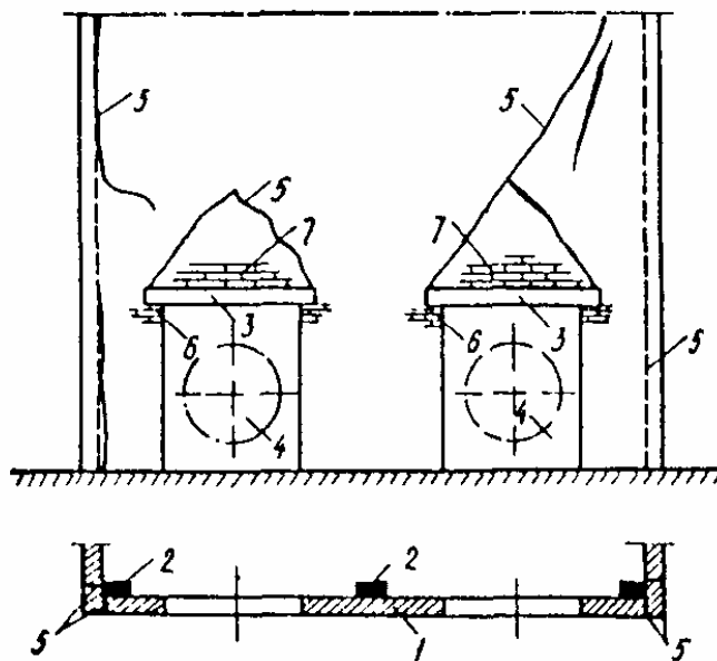
Рис. 20. Повреждение кирпичных стен при динамических воздействиях 1 - стена; 2 - колонна; 3 - перемычка; 4 - источник вибрации; 5 - трещина; 6 - разрушение кладки опор; 7 - расслоение кладки
