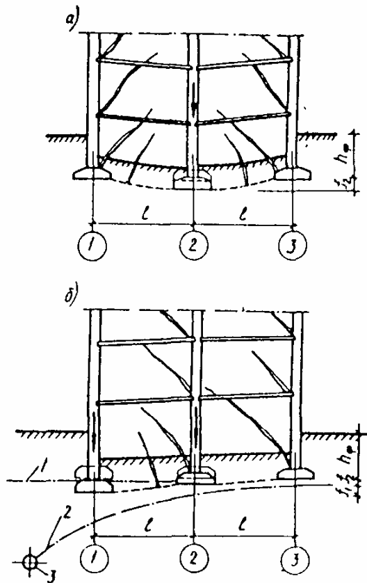
Рис. 19. Деформации и развитие трещин в поперечных стенах здания а - при просадке фундамента средней стены; б - при осадках фундаментов стен вследствие понижения уровня грунтовых вод при дренаже 1 - уровень грунтовых вод до дренажа; 2 - то же, после дренажа; 3 - дренажная труба
