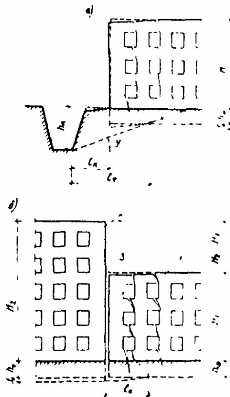
Рис. 18. Деформации и развитие трещин в стенах зданий а - при отрытии траншеи или котлована вблизи здания при l_k < l_\phi + 1 м; б - при пристройке нового здания большей высоты ( H_2 > H_1 ) 1 - старое здание; 2 - новое здание; 3 - осадочный шов
