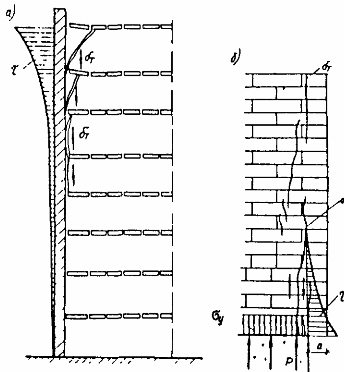
Рис. 12. Образование трещин сдвига (среза) \delta_m в стенах а - в местах сопряжения разнонагруженных (разнодеформируемых) стен; б - в местах нависания кладки ( a ); \tau - касательные; \sigma_y - нормальные напряжения
