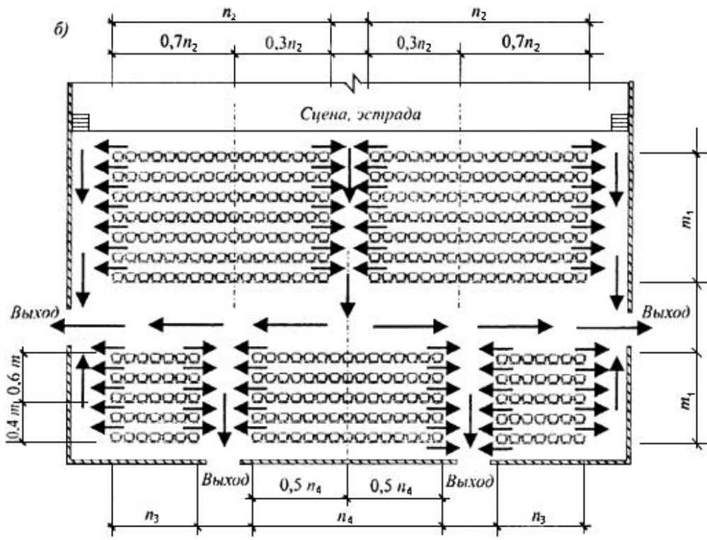
а - с боковыми (продольными) проходами; б - с поперечным проходом
